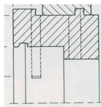
Zijaanzicht, montagevlak
